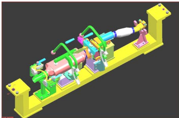
Beispiel: Prüfvorrichtung einer PKW-Abgasanlage
